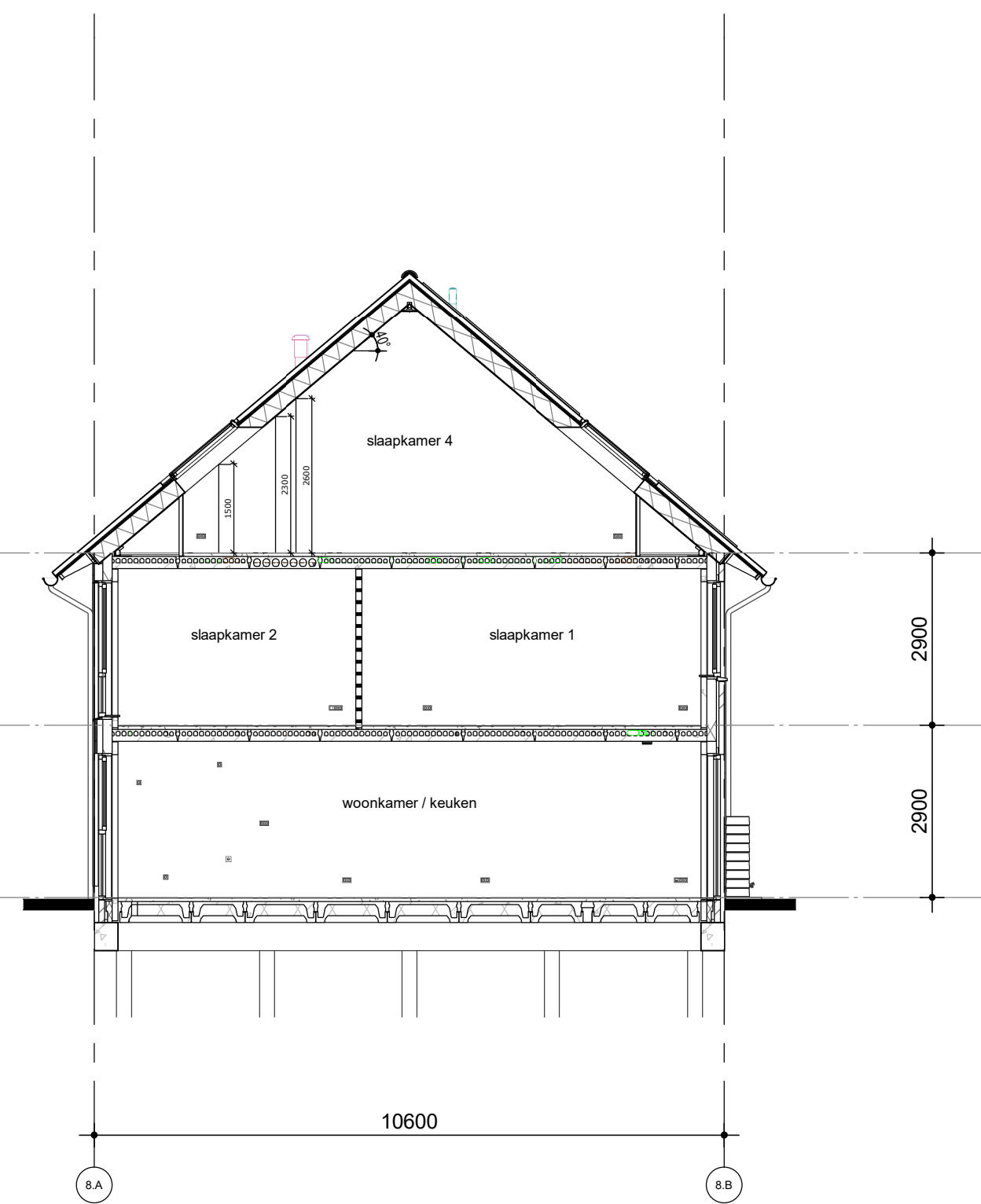
DOORSNEDE A 1 : 100
