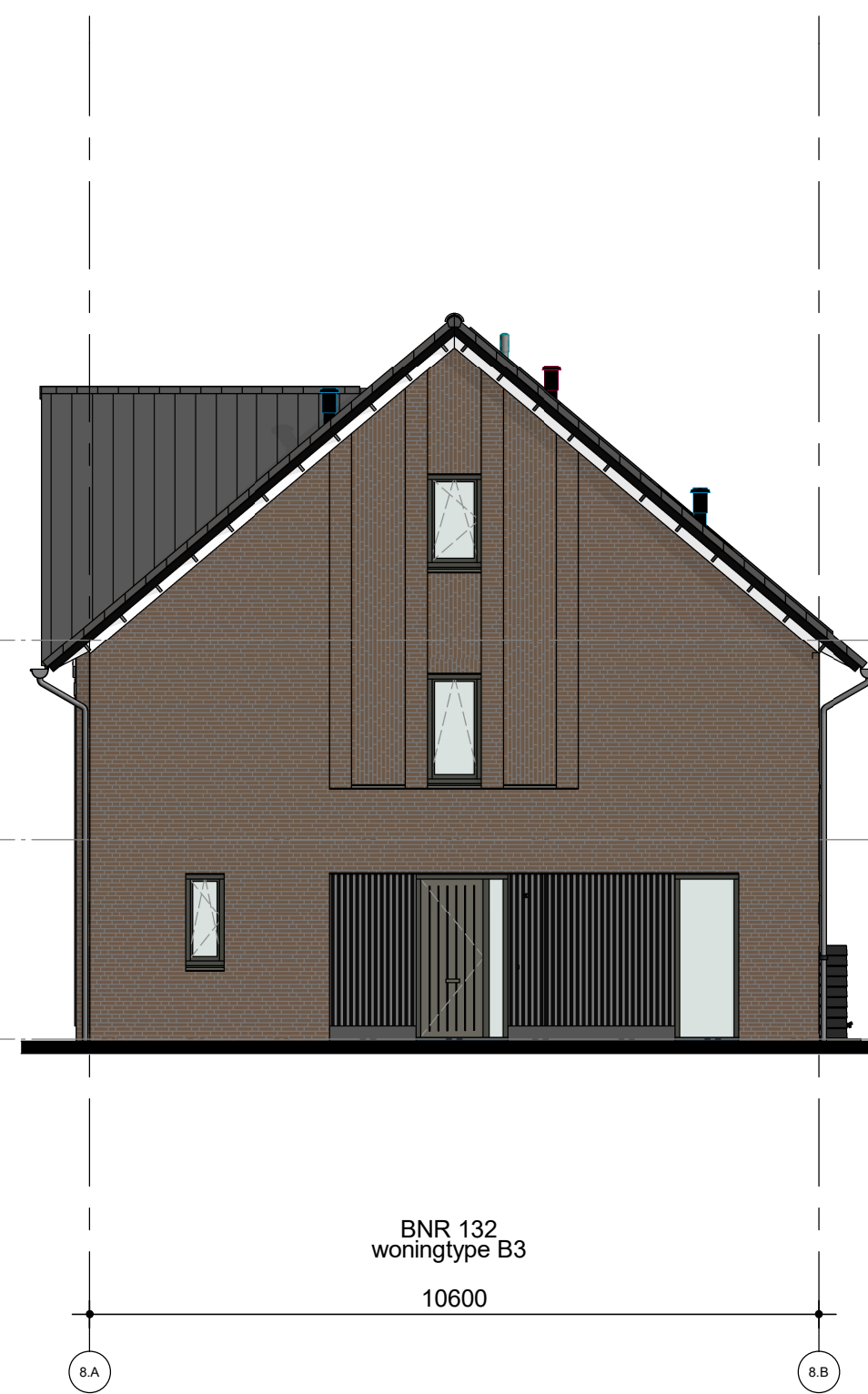
RECHTER ZIJGEVEL 1 : 100
