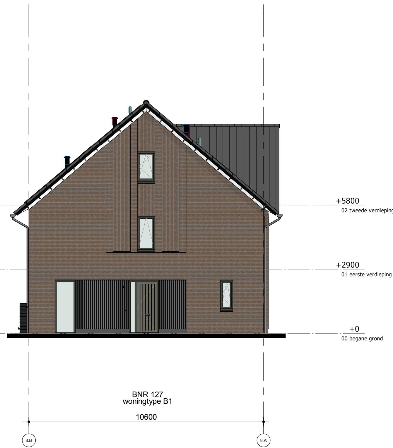
LINKER ZIJGEVEL 1 : 100
