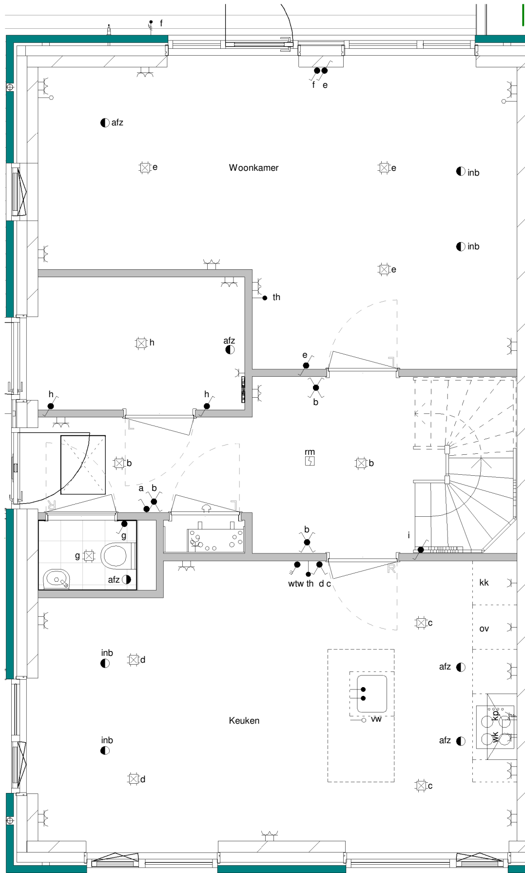
Begane grond R595 1 : 50
