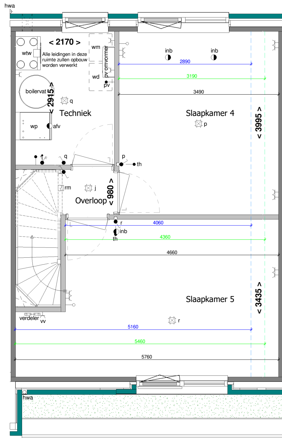
2e verdieping 1 : 50
