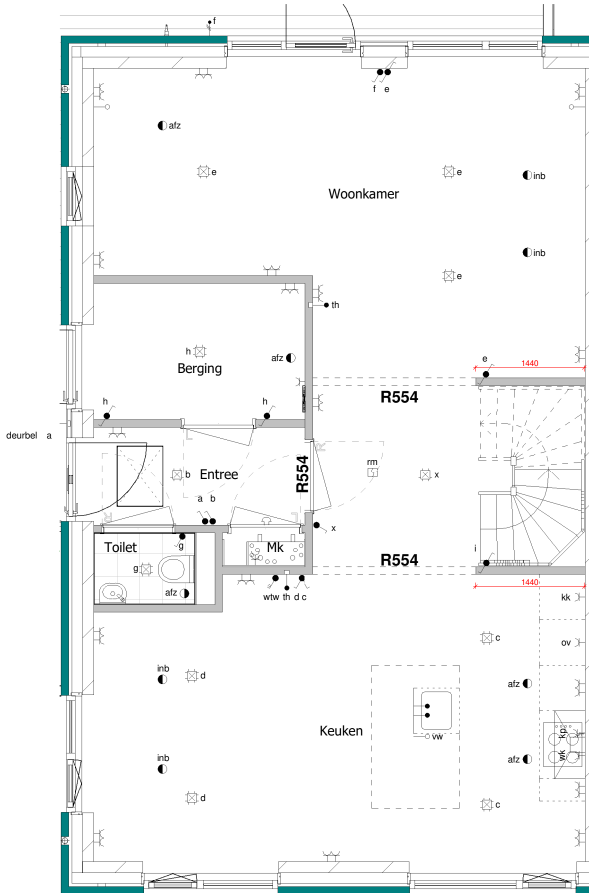
Begane grond R554 1 : 50
