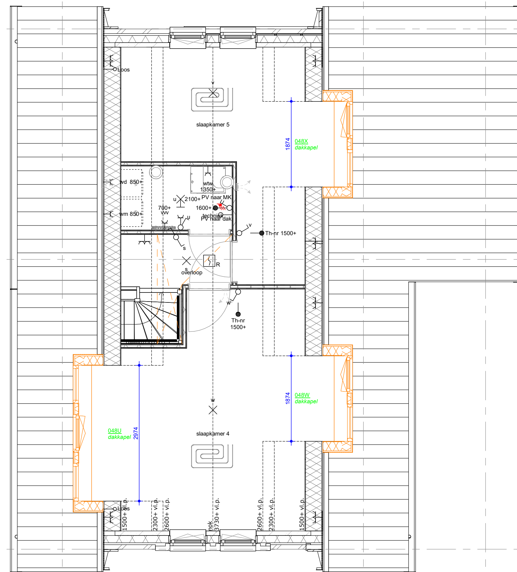
2e VERDIEPING
