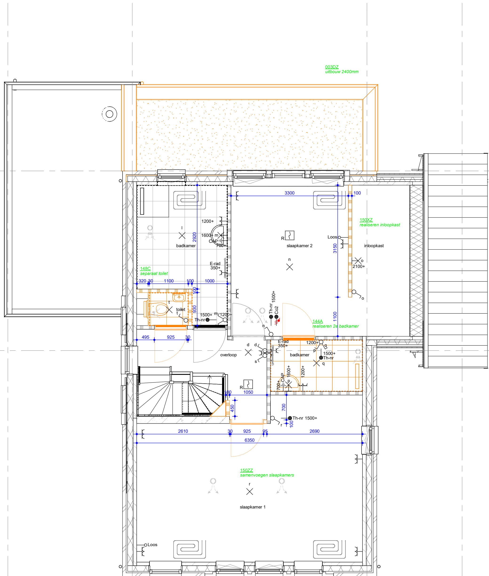
1e VERDIEPING
